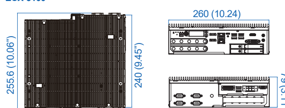
ECX-3100
