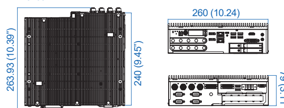
ECX-3200
