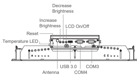
Left I/O
