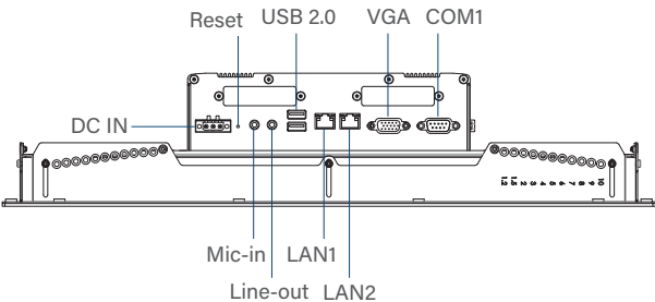
Right I/O
