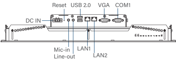
Right I/O
