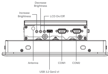
Left I/O
