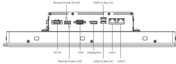
Right I/O
