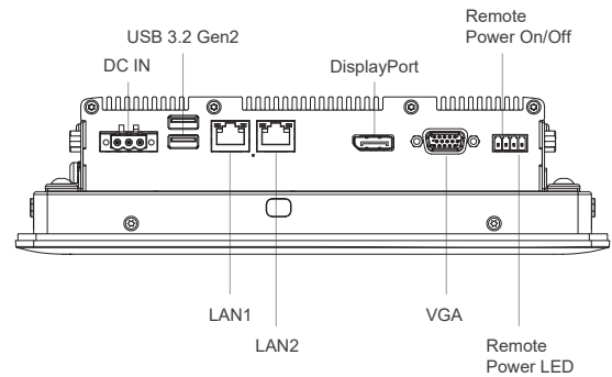
Right I/O
