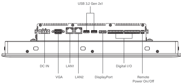
Right I/O
